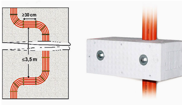
Bild 4: Möglichkeiten der Verlegung in Steigzonen, mäandernd oder mit WUM.
