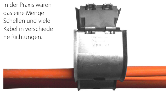
Bild 3: Hermannschelle von Dätwyler IT Infra.
