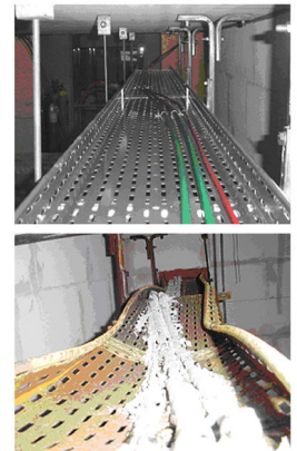
Bild 1: Funktionserhaltprüfung von Kabelanlagen im Brandofen – vorher und nachher.
