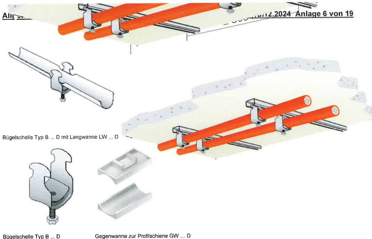
Bügelschelle Typ B ... D
