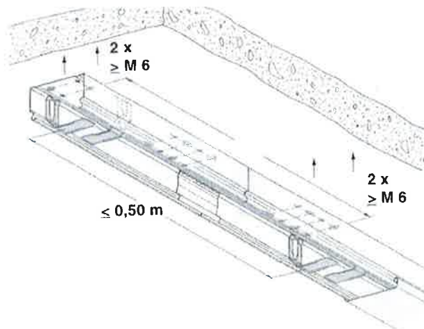
Deckenmontage
