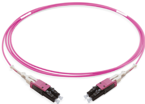
Cavo patch DCS (FR/LSZH), 2 fibre OM4
