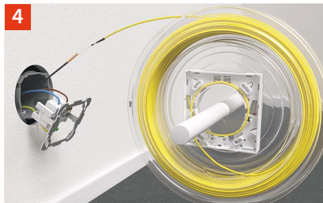
Mit einer Stange (oder ähnlichem) das LWL-Kabel locker abrollen und das Kabel einziehen.
