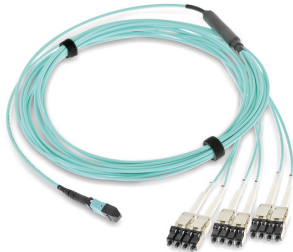
FO-DCS Fanout-Kabel, MTP-auf-LCDU, 12 Fasern
