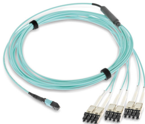
FO-DCS fanout kabelk, MTP-op-LCDU, 12 vezels
