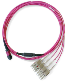
Câble FO-DCS fanout MTP-sur-LCDU, 8 fibres
