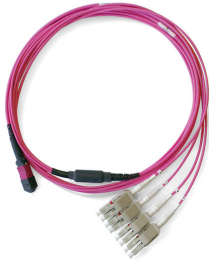
FO-DCS fanout-kabel, MTP tot LCD, 8 vezels
