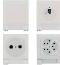
Anwendungsbeispiele: mit Blinddeckel, mit TT83, mit TV und mit 3x Typ 13
