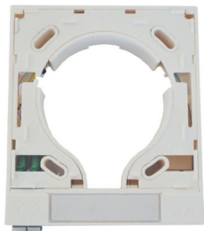
Salida de datos de FTTH Squeeze AP, 88 x 112 x 19 mm
