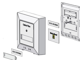
Ensemble OTO Cover-AP pour les rénovations des prises OTO existantes, blanc
