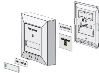
AP Cover-Kit zum Nachrüsten bestehender OTO-Dosen, weiss
