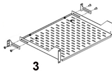
3. Étagère 2U avec des fixations pour le renfort standard
