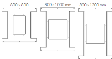
Ontwerp bovenplaat
